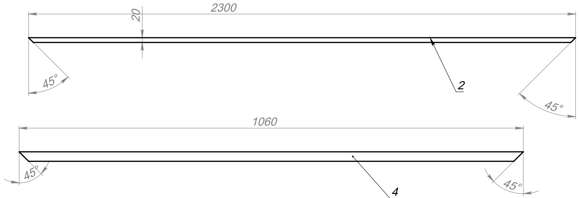
A-A (1 : 20)
